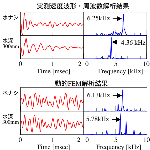
図 3 実測および動的 FEM 解析結果
