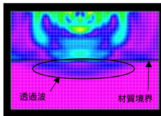
図 4 動的 FEM 解析による縦弾性波の挙動
